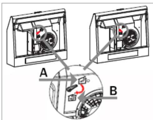
A: Tryb wyciągu (wentylacja powietrzem zewnętrznym)
